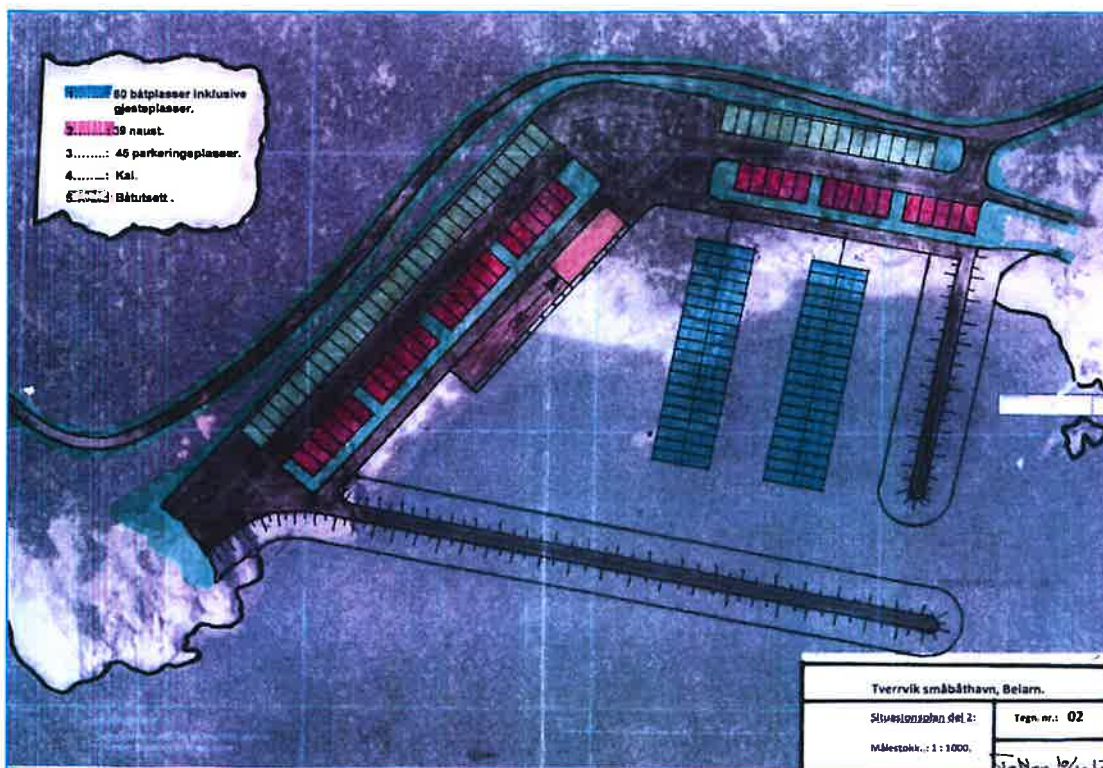
Figur 6. Skisser som viser utkast til løsning for småbåthavna med landdel. Kilde: Ingeniør Terje Nordland.
